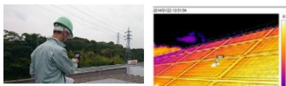
サーモグラフィによるパネル温度測定
